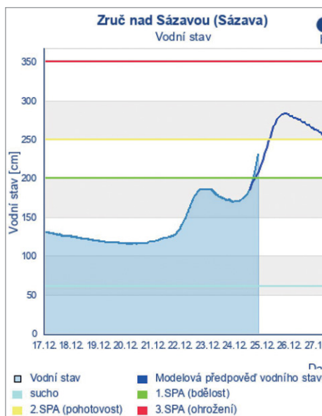
Modelová předpověď vodního stavu z 24. 12. 2023 pro Zruč nad Sázavou
